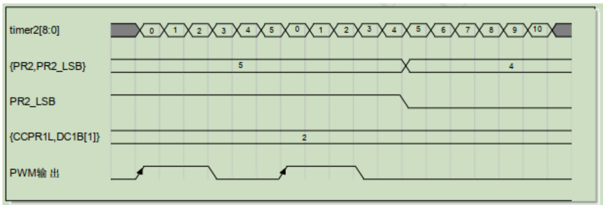
图 1-1 错误清零 PR2_LSB 导致 PWM 输出错误的时序图 (T2RES=0)
